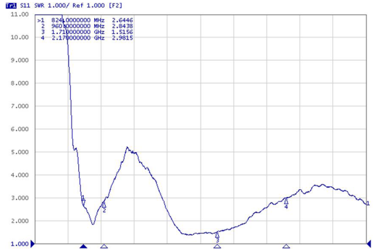
VSWR
